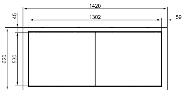
Boven aanzicht
